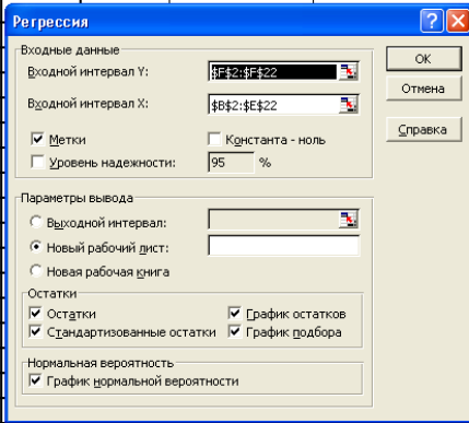
Рис.4. Диалоговое окно Регрессия подготовлено к выполнению анализа данных Результаты обработки данных с помощью инструмента регрессия представлены ниже в таблицах 3 -6.
